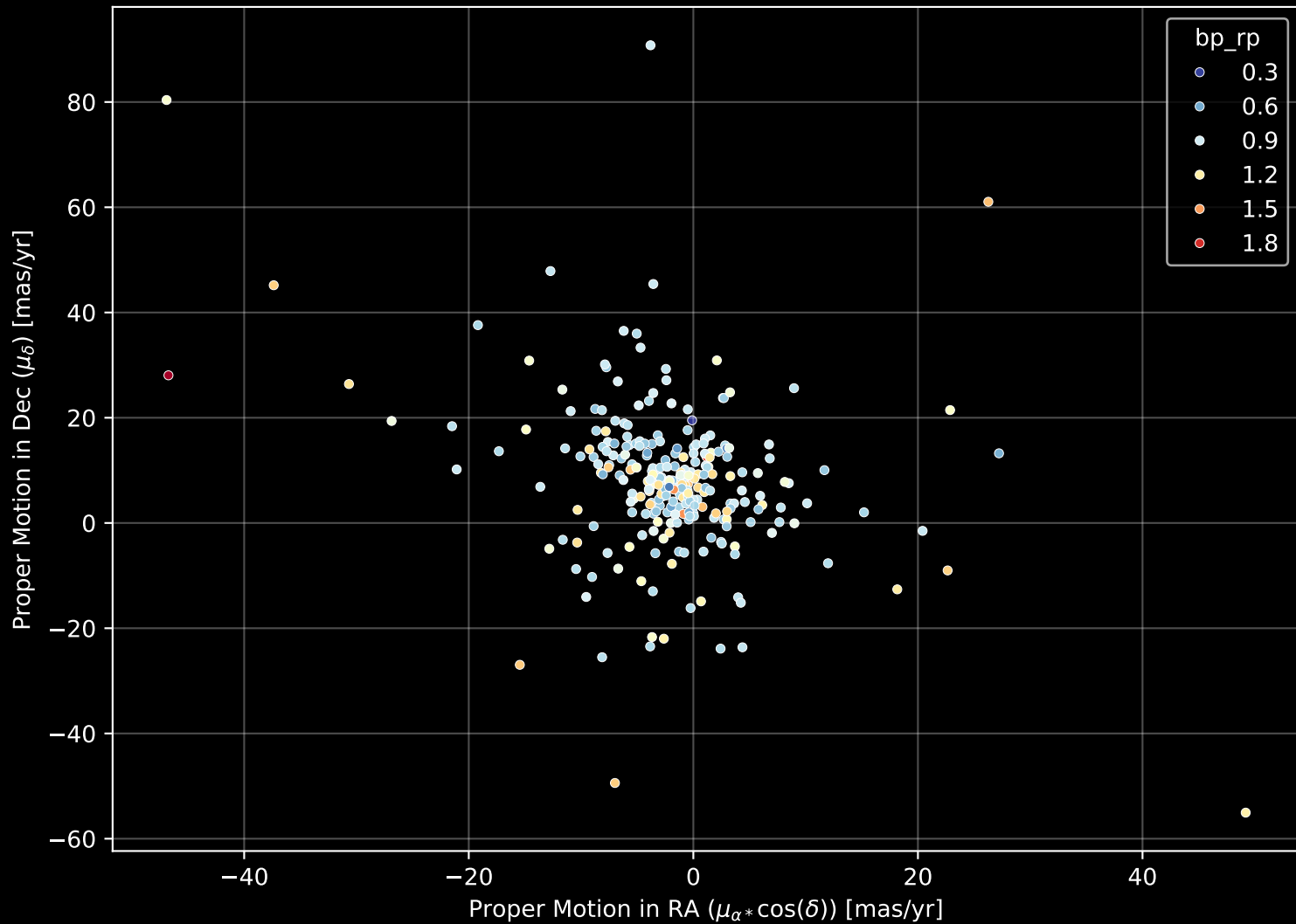
GALAH DR4 Field: [2057] Proper Motion Diagram (n= 273)
