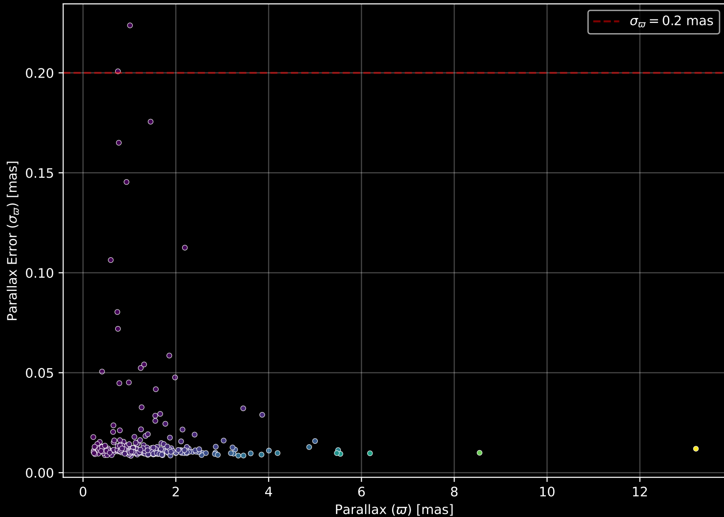
GALAH DR4 Field: [2057] Parallax Quality (n= 273)
