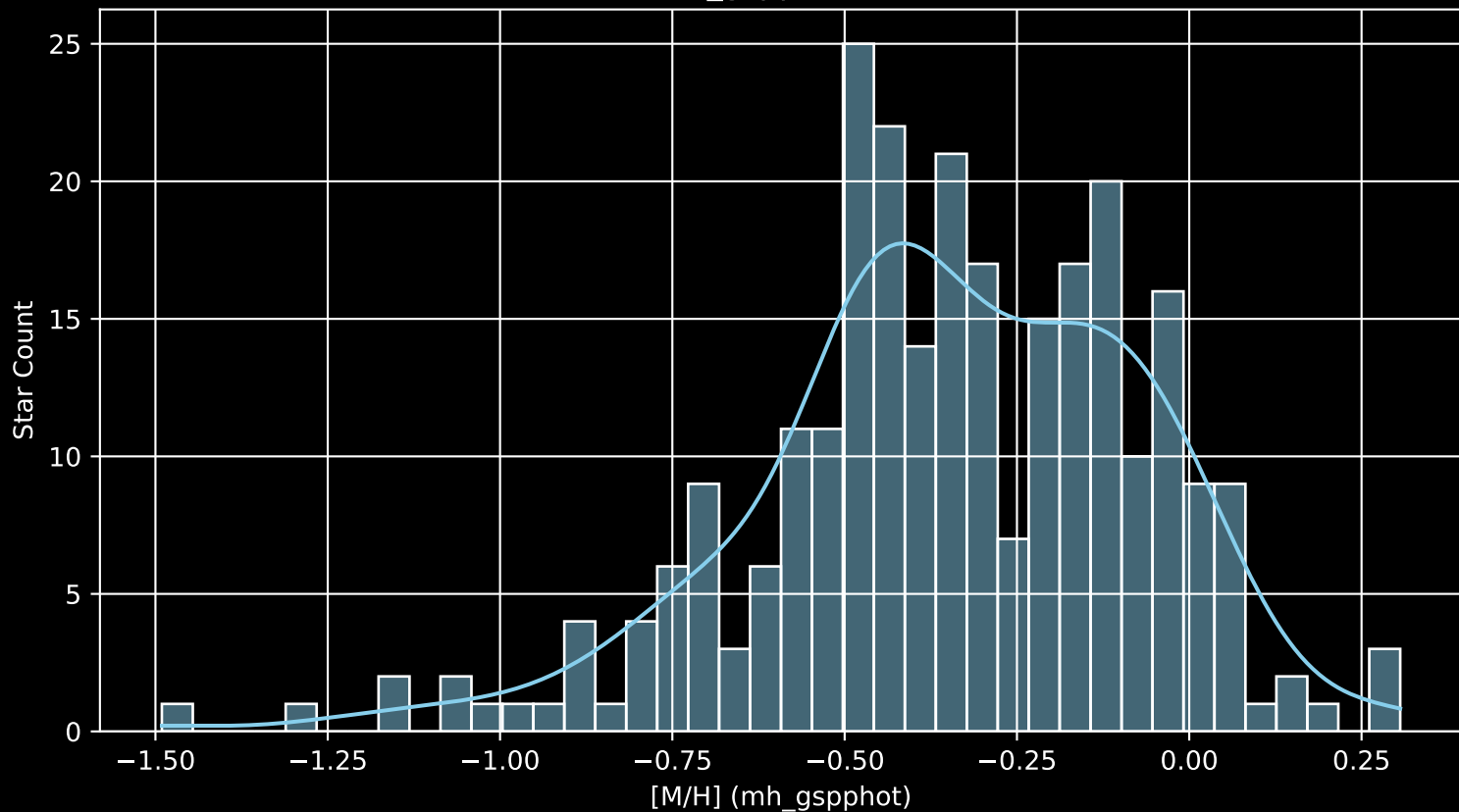
GALAH DR4 Field: [2057] [M/H] (mh_gspphot) (n= 273)
