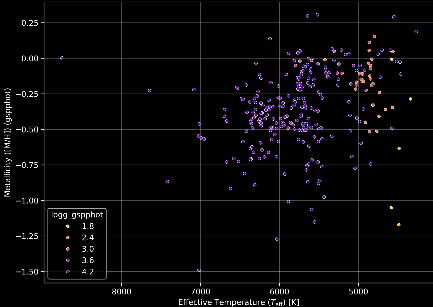
GALAH DR4 Field: [2057] Stellar Population Parameters (n= 273)
